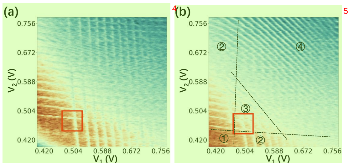
图 3.11 自动调控的结果。(a) 自动调控前双量子点的电荷稳定图。(b) 自动调控后双量子点的电荷稳定图。其中①②③④分别为无点区，单点区，适中耦合的双点区和过耦合的双点区。 6
