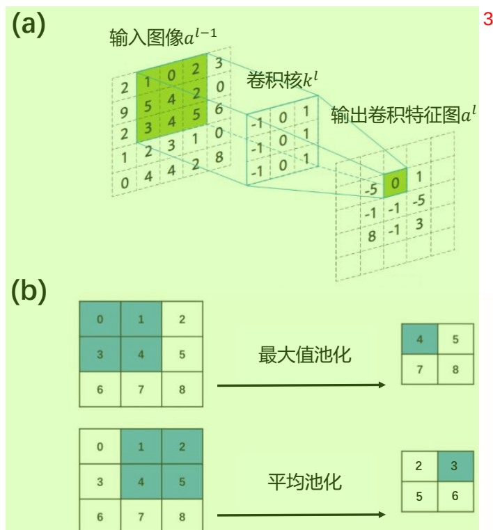
图 2.1 卷积和池化过程。(a) 卷积操作。输入的图像经过卷积核后得到输出特征图，且长度和宽度减少量等于卷积核长宽减 1。 3 (b) 池化操作。在平均池化中将选中区域求平均值并输出，在最大值池化中取选中区域的最大值并输出。 4
