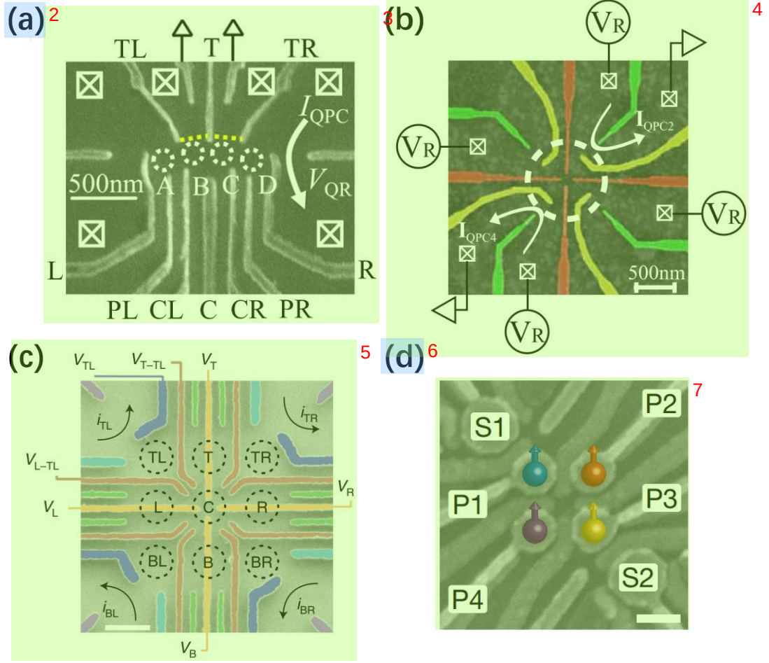
图 4.1 几种不同的量子点阵列结构。(a) 线性阵列结构。(图片引自文献[13])。(b) 闭合路径阵列结构。(图片引自文献[14])。(c) 二维 3 \times 3 阵列结构。(图片引自文献[16])。(d) 矩形阵列结构。(图片引自文献[15])。 8
