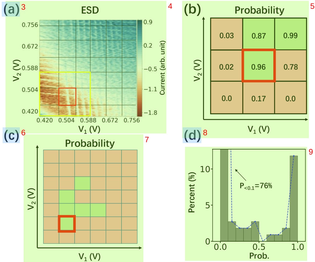
图 3.9 少电子区的搜索过程。(a) 双量子点的电荷稳定图。在处理过程中相图按照约 0.06 \text{ V} \times 0.06 \text{ V} (31 px) 的大小被划分为多个部分,在此例中相图被分为 42 个部分,每一个部分将分别由 CNN 进行识别并分类。(b) CNN 给出的电荷稳定图中各区域处于双点状态的概率。图中给出了一部分详细的概率值,概率值高于 80% 的部分被记录为双点态,低于 80% 的部分被记录为非双点态,分别使用绿色和红色标注。(c) 完整电荷稳定图中由 CNN 给出的各区域处于双点态的概率。少电子区通过选取概率高于 80% 的区域中拥有最低电压的部分进行定位。结果由红色框标注。(d) 相图中电荷态识别的概率分布直方图。
