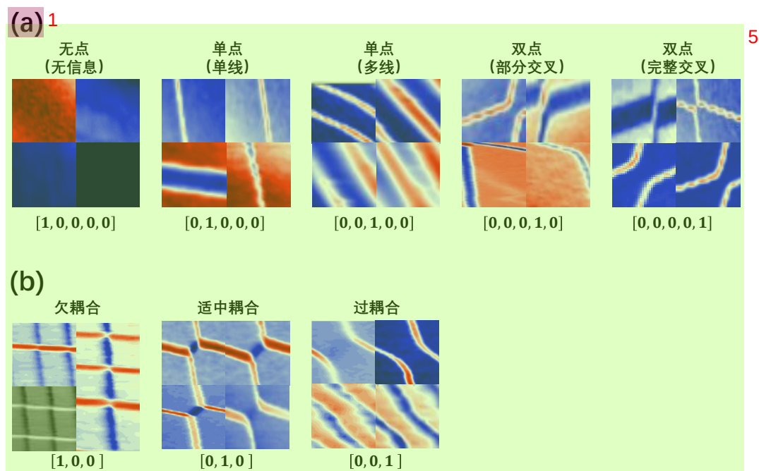
图 2.7 用于神经网络训练过程的相图样本以及对应的标签。(a) 用于训练寻找少电子区的神经网络的样本示例。(b) 用于训练判定耦合强度的神经网络的样本示例。
