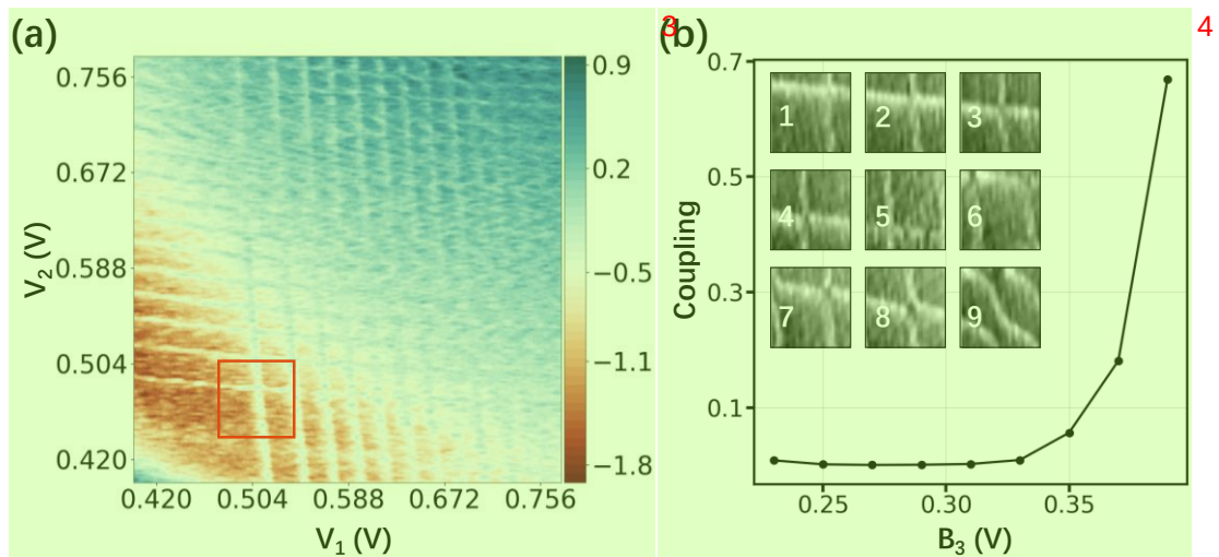
图 3.10 对量子点间耦合的调控过程。(a) 双量子点的电荷稳定图。在耦合调节过程中仅针对红色方框区域进行相图测量。(b) 基于 CNN 的耦合调控过程。调节顺序按照 1~9 进行，其势垒电极电压按照 0.02 V 的步长从初始的 0.23 V 被调节到 0.39 V。相图下方的数字为 CNN 耦合识别的返回结果，表示对应相图所属的类别。
