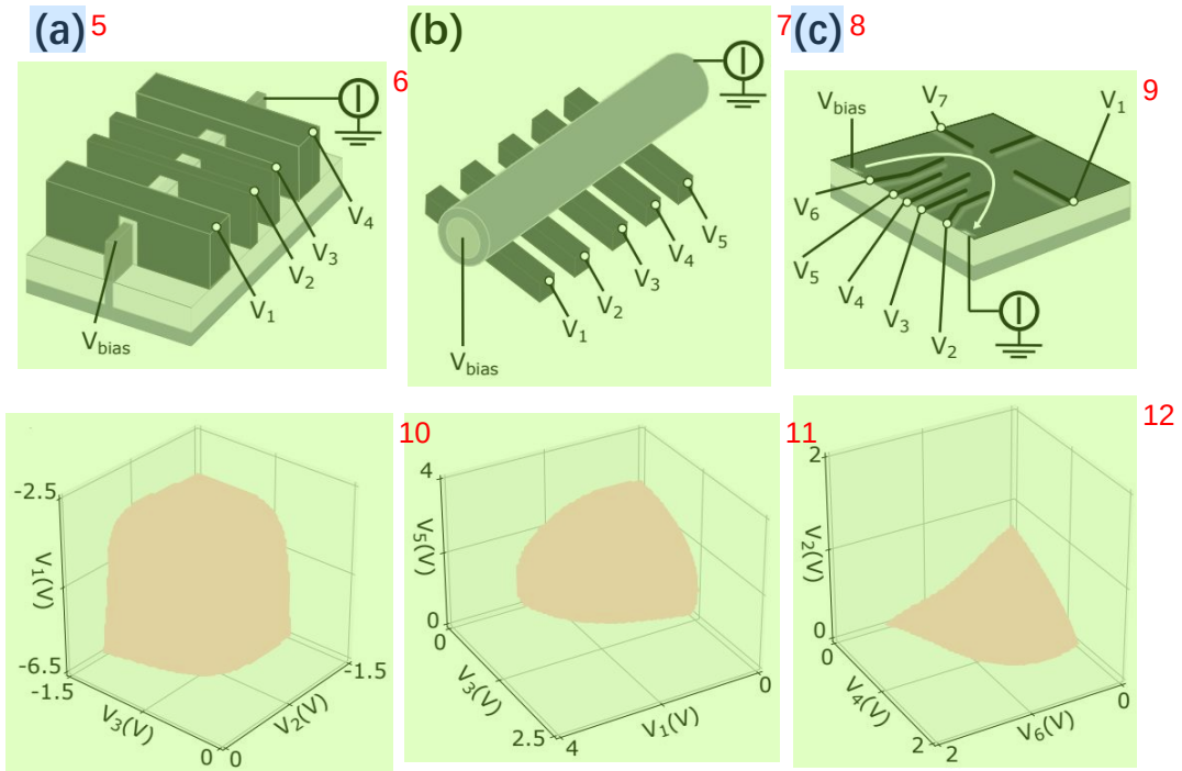
图 1.6 多量子点系统的输运图像。(a) 硅基 FinFET 量子点器件结构示意图以及三维电荷稳定图。(b) 硅锗纳米线器件结构以及对应的电荷稳定图。(c) 硅锗异质结器件结构以及对应的电荷稳定图。(图片引自文献 [29] )
