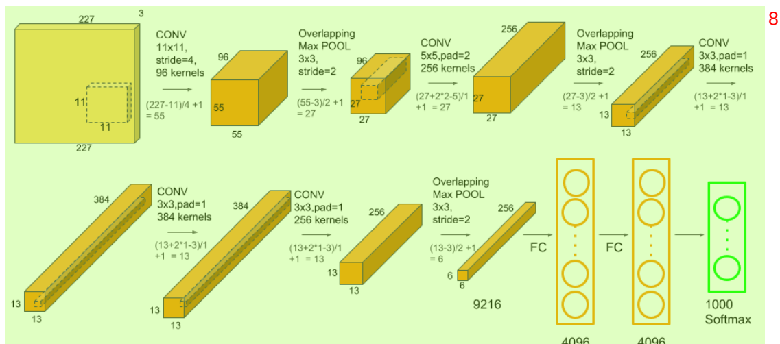
图 2.2 AlexNet 网络结构示意图。网络中包含 5 个卷积层，3 个池化层以及 3 个全连接层。 9 （图片来自网络）
