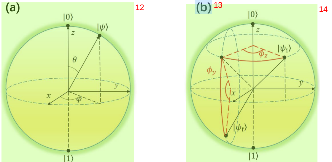
图 1.1 布洛赫球示意图。(a) 定义量子比特的布洛赫球。其中 |0\rangle 和 |1\rangle 分别代表两种量子态在球面上的位置，球的半径为 1，表示系数的归一化， |\psi\rangle 表示量子比特的量子态，其在球面上任意一点都可以用极角 \theta 和方位角 \varphi 表示。(b) 在球面上展示的单量子比特操作。从初始态 |\psi_i\rangle 到达末态 |\psi_f\rangle 的过程可通过绕 z 轴转动角度 \phi_z 以及绕 y 轴转动角度 \phi_y 实现。(图片引自文献[11]) 15
