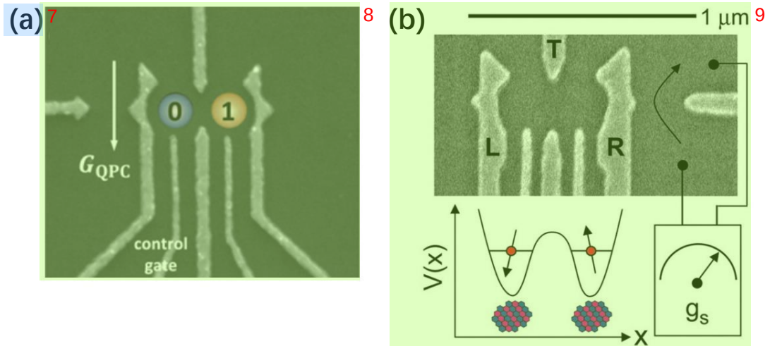
图 1.2 电荷量子比特和 S-T 量子比特。(a) 电荷量子比特通过单电子电荷在左或右量子点中的位置来编码信息。(b) 利用双电子自旋态定义的 S-T 量子比特。(图片引自文献[20]) 10
