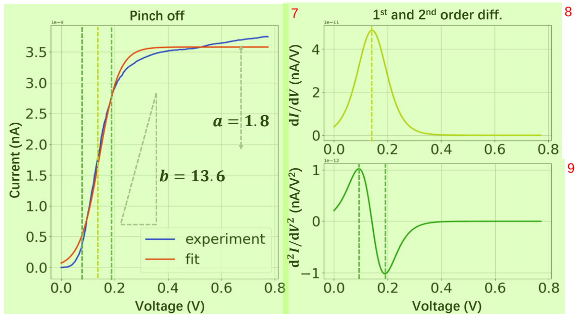
图 3.7 夹断电流曲线及其拟合曲线。曲线的最大斜率的位置以及两个拐点的位置分别通过计算一阶和二阶导数获得。 10
