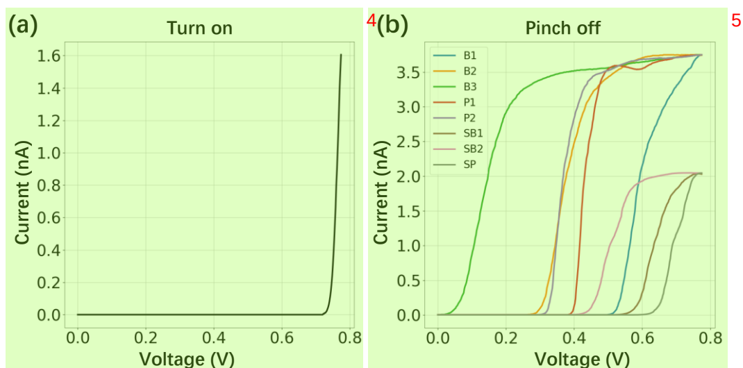
图 3.2 开启和夹断电流测试。(a) 量子点的开启电流。横坐标的电压表示所有栅极的同时 6 改变。(b) 量子点的夹断电流。不同的曲线分别代表不同的栅极。
