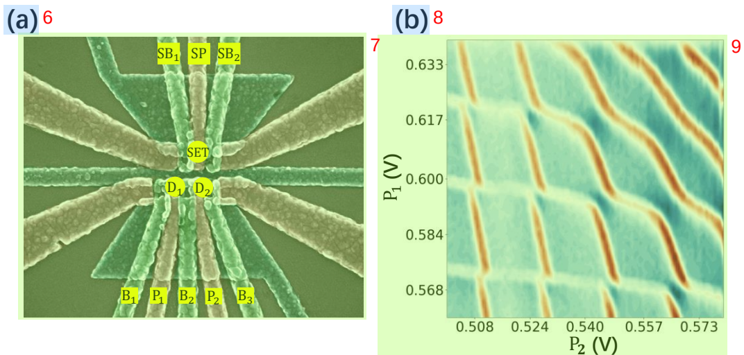
图 3.1 (a) 双量子点的电镜图 (已上色)。(b) 调控后的电荷稳定图。
