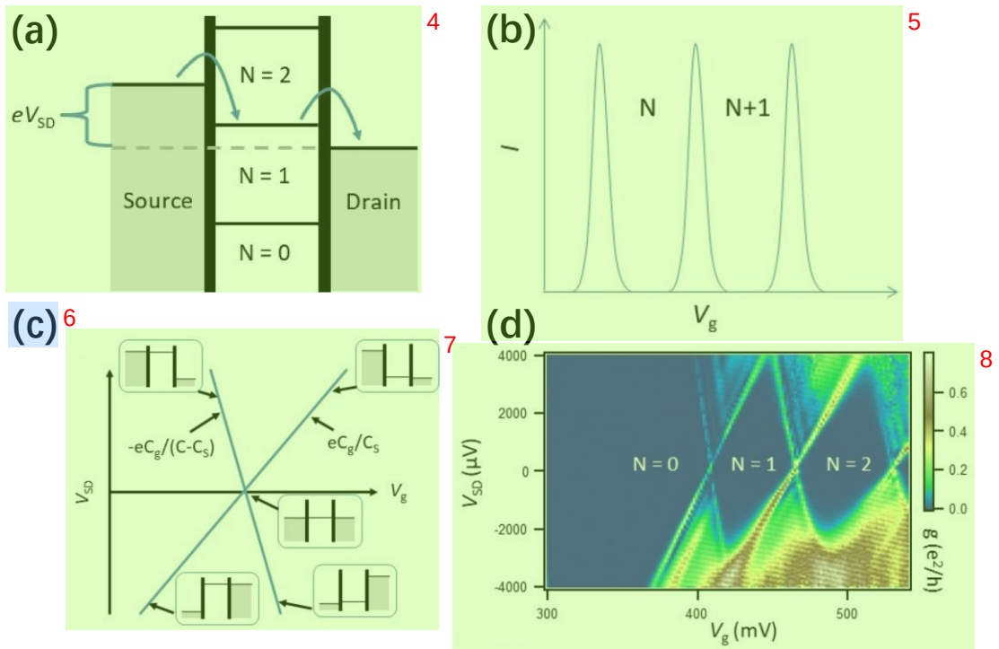
图 1.4 单量子点输运示意图。(a) 通过对源漏施加偏压 V_{SD} 产生势能差，电子在电场的作用下产生输运的过程。(b) 当栅极电压 V_g 发生改变引起量子点中电化学势变化时，会观察到库仑振荡现象。(c) 库仑菱形示意图。正斜率直线表示量子点能级与漏极费米面持平，负斜率直线表示量子点能级与源极费米面持平。(d) 实验中观测到的库仑菱形。(图片引自文献 [14] )
