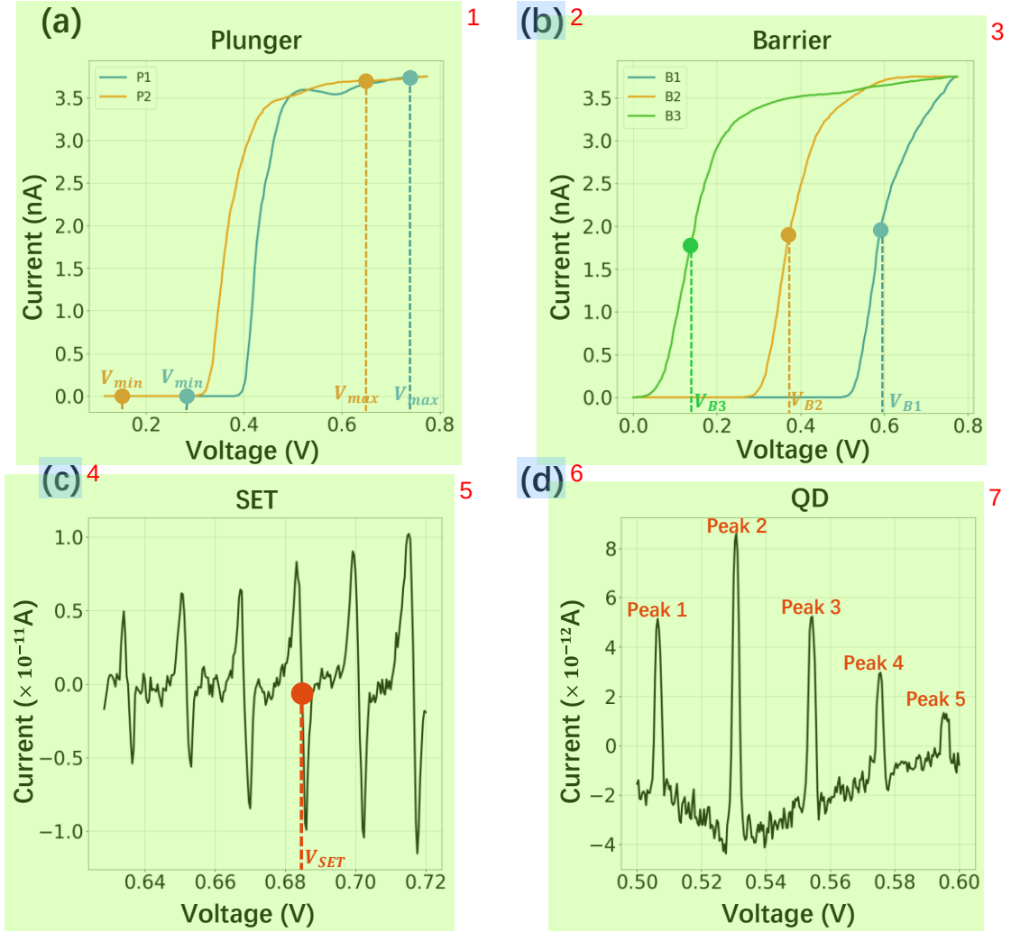
图 3.3 对量子点的初步表征。(a) 通过扫描泵浦电极电压的夹断曲线确定其大致的工作范围 8 。P1 和 P2 栅极的电压范围分别用蓝点和橙点在图中标出。(b) 通过扫描势垒电极电压的夹断曲线确定其初始电压位置。三个势垒电极 B1、B2 和 B3 对应的初始电压分别由蓝点、橙点和绿点在图中标出。(c) 通过扫描 LP 栅极确定 SET 的工作电压。其中 SET 随电压响应最敏感的位置由红点在图上标出。(d) 通过扫描 P1 (或 P2) 栅极确认量子点的成点情况。在图中展示出了 5 个振荡峰，每个振荡峰都代表电子进出量子点的过程。顺利形成振荡峰意味着量子点可以正常工作。
